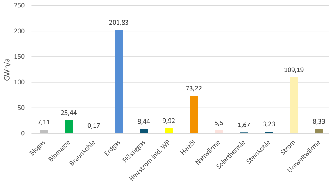
Abbildung 19: Endenergieverbrauch nach Energieträgern 2021
