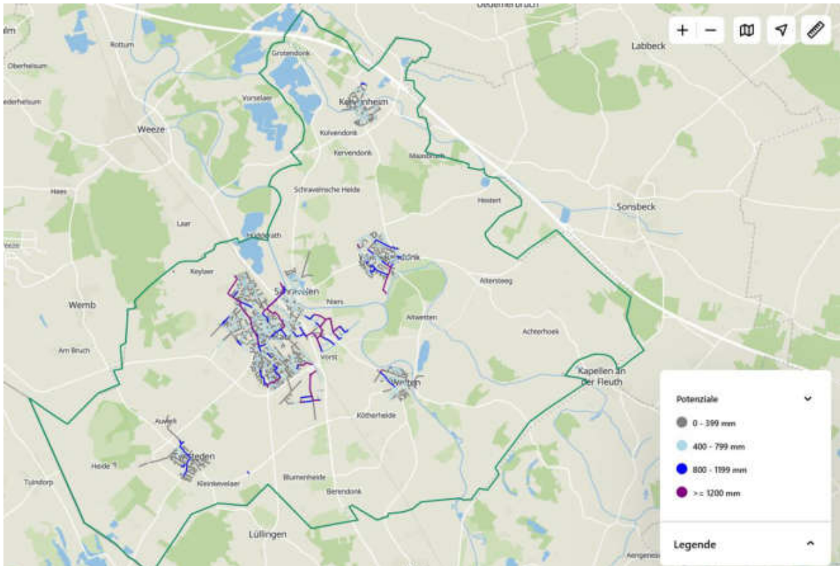
Abbildung 37: Abwassernetz Kevelaer, aggregiert nach Nennweiten der Kanäle. Quelle: digitaler Zwilling (digipad)
