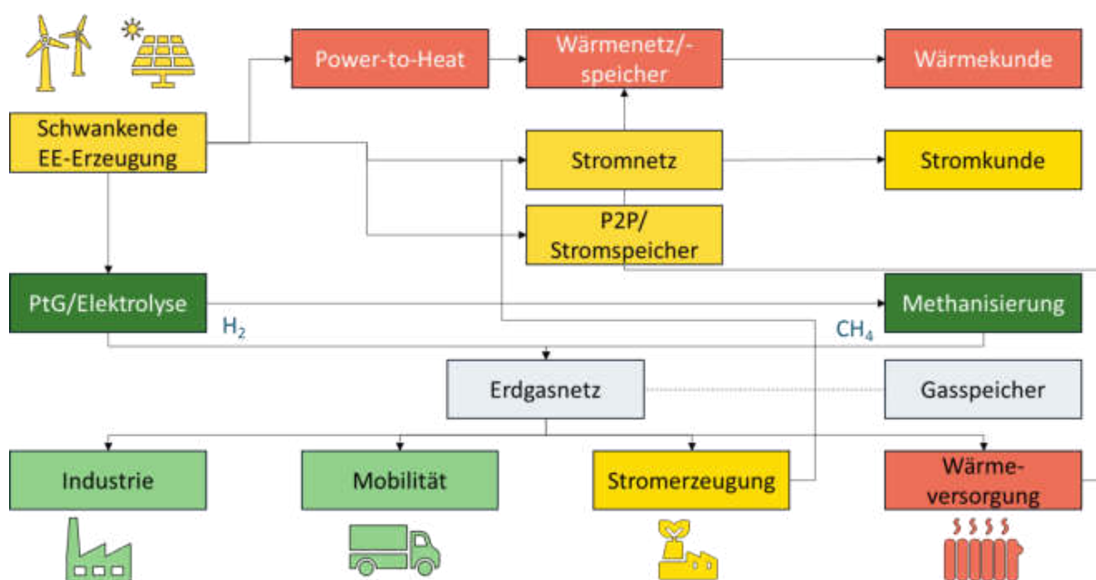
Abbildung 65: Übersicht verschiedener Power-to-X Prozesse
