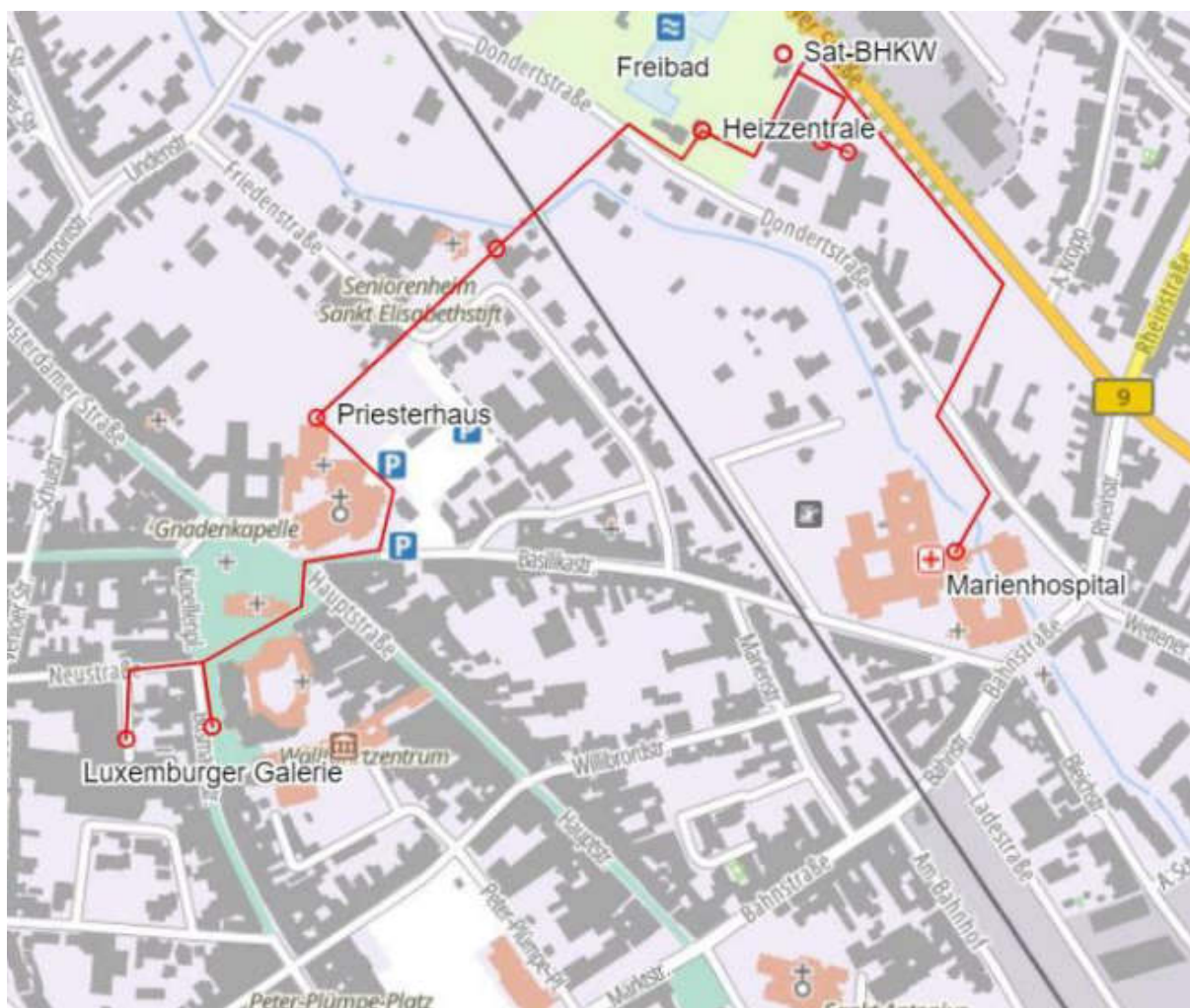
Abbildung 61: Trassenverlauf des Gebäudenetzes in Kevelaer. Quelle: Schloss Wissen
