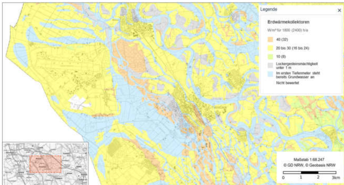
Abbildung 44: Geothermische Ergiebigkeit für Erdwärmekollektoren [7]
