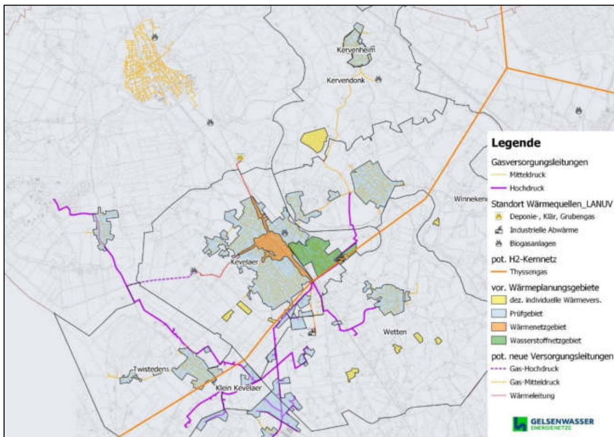
Abbildung 62: Gasnetztransmutationsplanung der Gelsenwasser Energienetze GmbH. Quelle: Gelsenwasser
