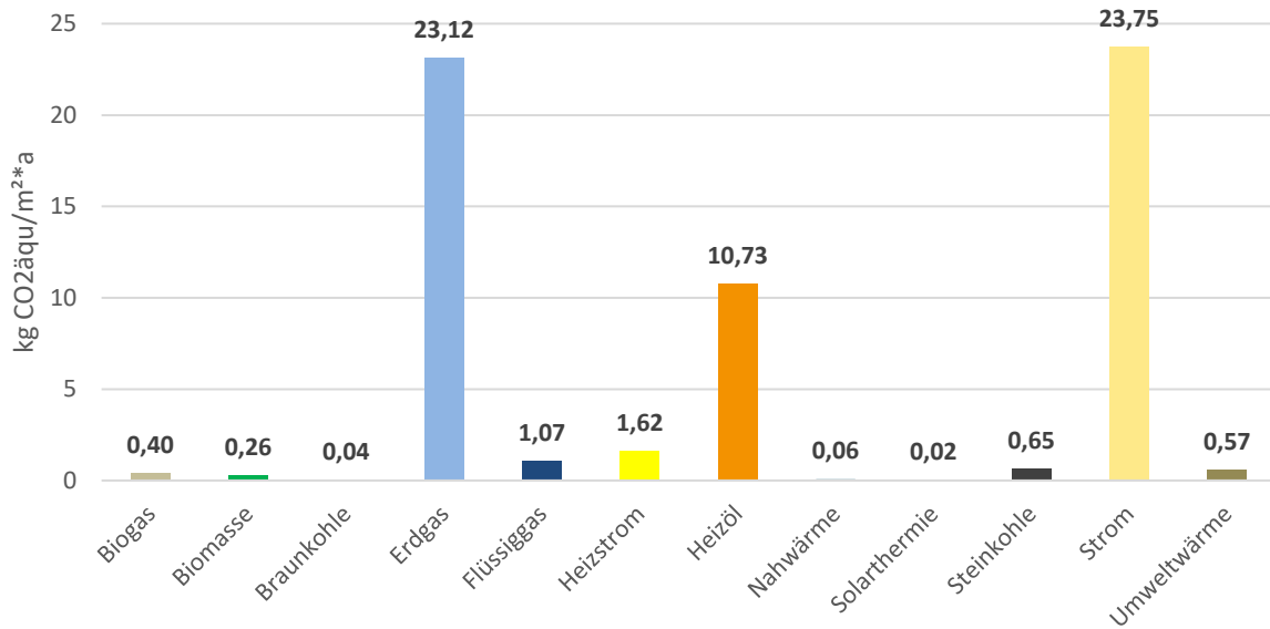
Abbildung 25: Aufteilung der THG-Emissionen für 2021 nach Energieträger
