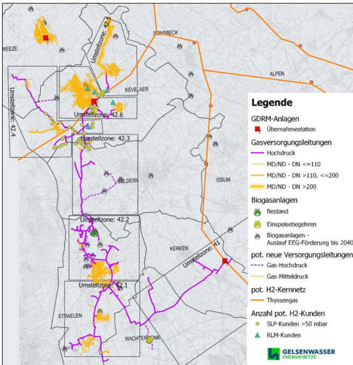
Abbildung 63: Potentialanalyse Wasserstoff gem. Gasnetztransformationsplanung der Gelsenwasser Energie-netze GmbH. Quelle: Gelsenwasser
