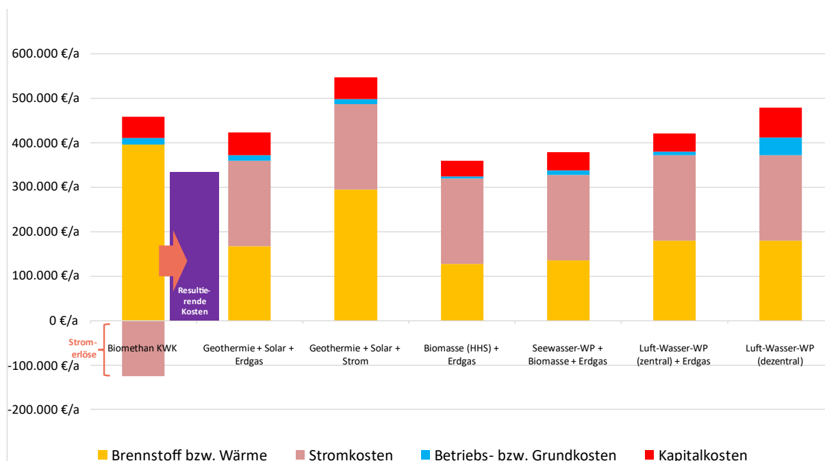
Abbildung 76: Vollkostenvergleich der Wärmeerzeugungsvarianten
