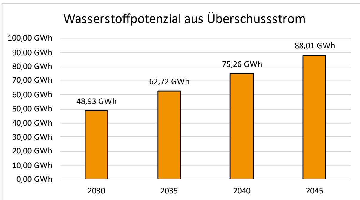
Abbildung 70: Theoretisches jährliches Wasserstoffpotenzial aus Überschussstrom EE für Elektrolyse
