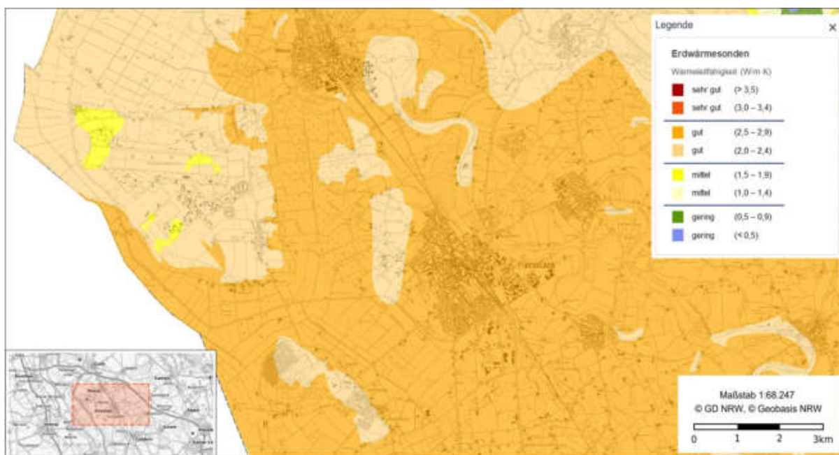
Abbildung 47: Geothermische Ergiebigkeit für Erdwärmesonden bei 40 m Tiefe [7]
