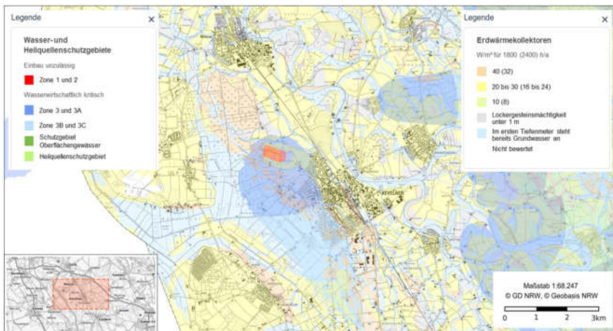
Abbildung 46: Wasserrechtliche Schutzgebiete in Kombination mit thermischer Ergiebigkeit [7]
