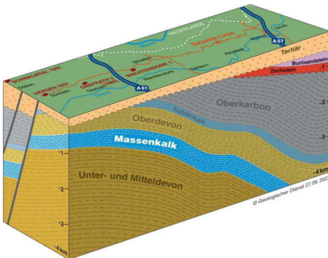
Abbildung 51: geologische Schichten in der Region. Quelle: [11]
