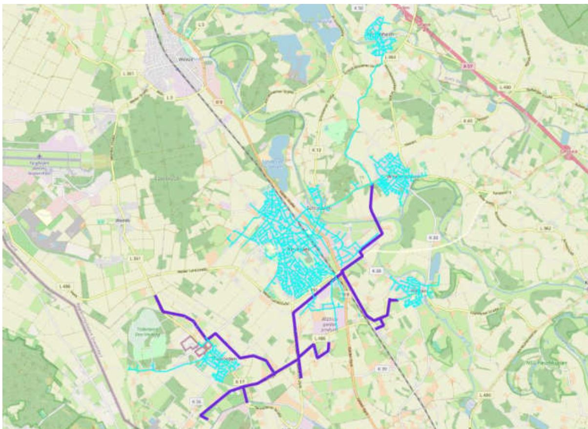
Abbildung 34: Transportleitungen (lila) und Verteilungen (blau) Gasnetz Kevelaer. Quelle: digitaler Zwilling (digipad)
