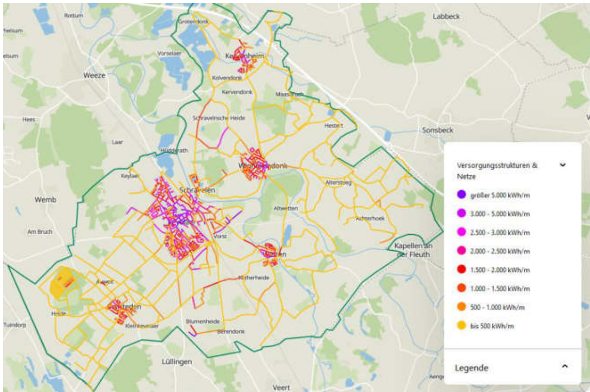
Abbildung 77: Wärmelinendichten im Planungsgebiet. Quelle: digitaler Zwilling (digipad)
