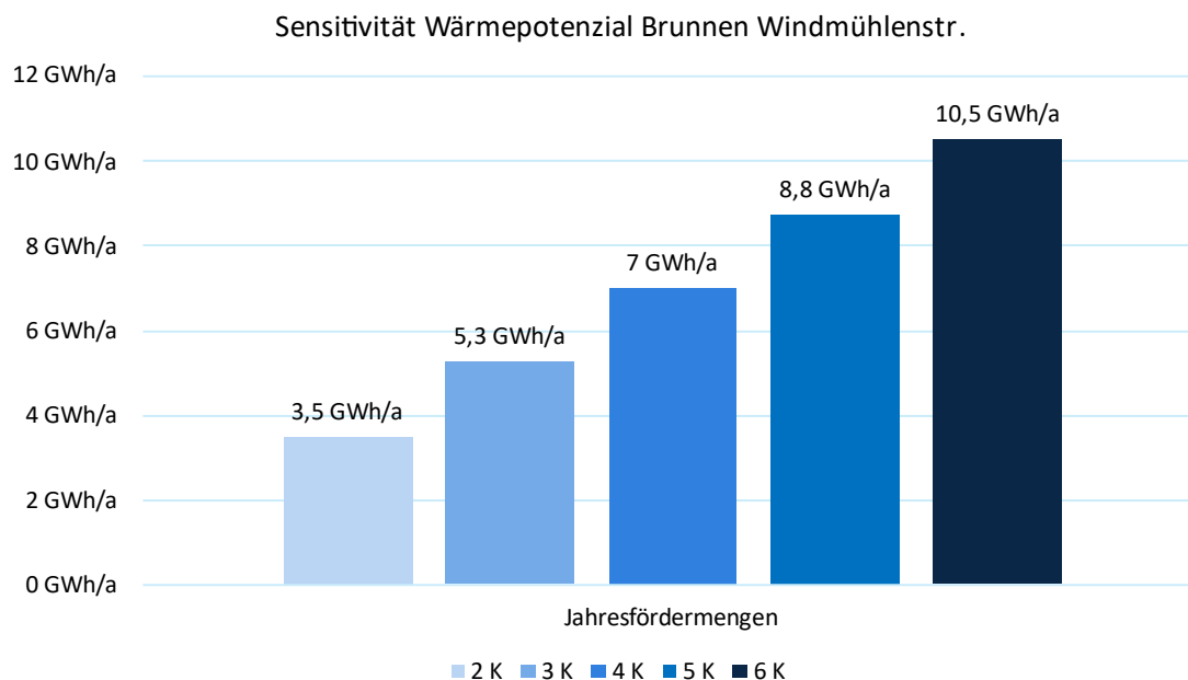
Abbildung 50: Wärmemengen für Grundwasserbrunnen Windmühlenstr. für versch. Temperaturabsenkungen des Grundwassers
