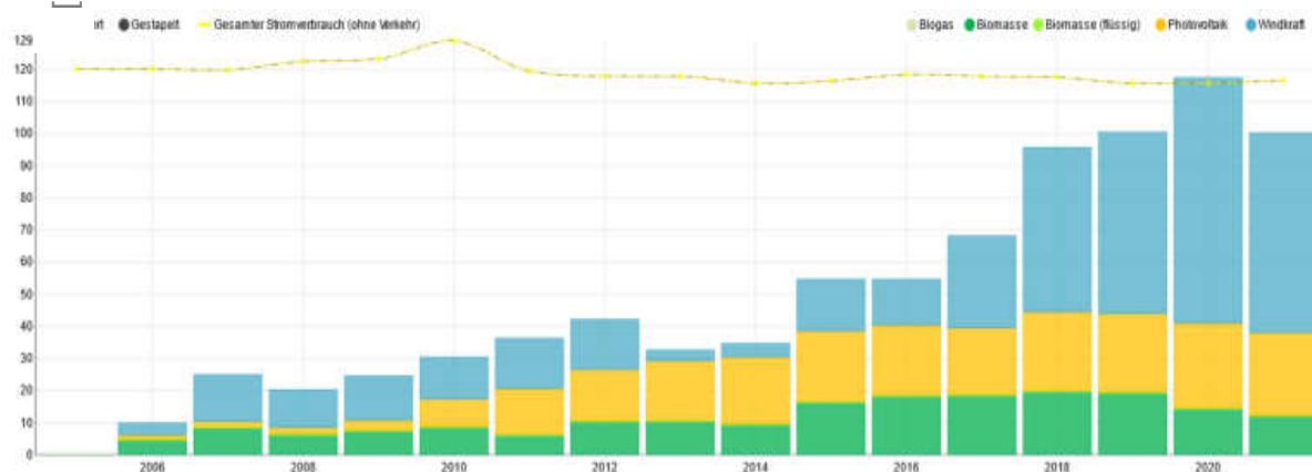
Abbildung 32: Bereitstellung von Strom aus lokalen EE-Anlagen
