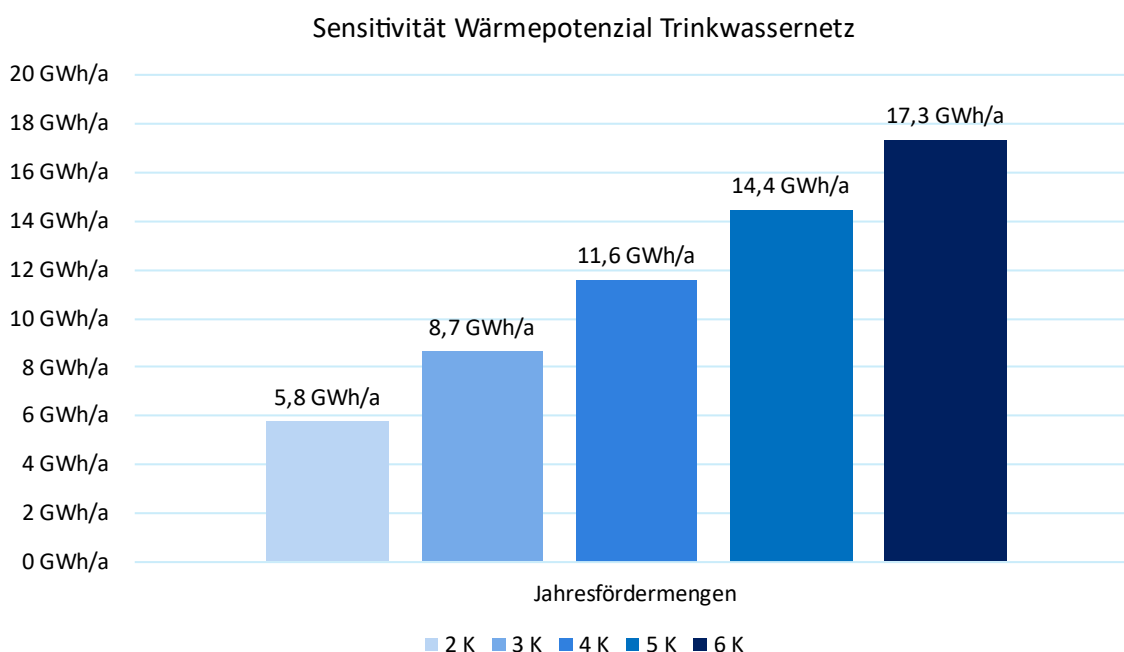
Abbildung 55: Mögliche Nutzwärmemengen einer Trinkwasser-Wärmepumpe in Abhängigkeit verschiedener Temperaturabsenkungen
