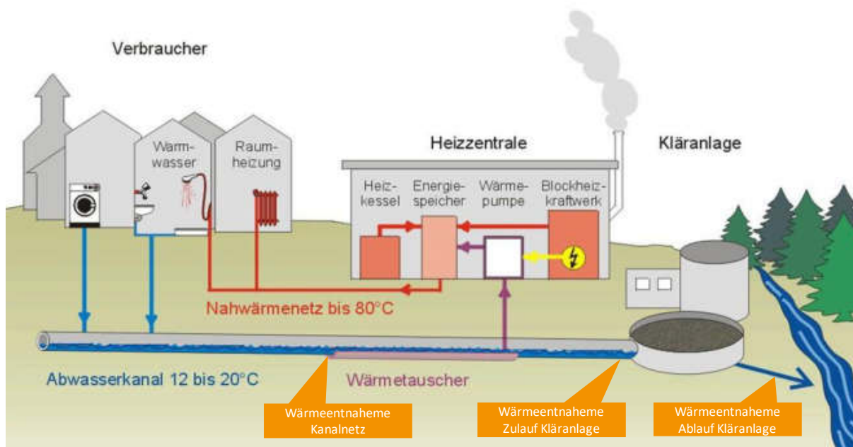
Abbildung 56: Technische Möglichkeiten des Wärmeentzugs aus Abwasser [12]
