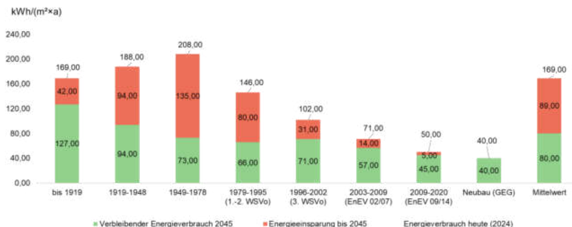
Abbildung 40: Flächenbezogener Endenergieverbrauch für Wohngebäude nach Altersklasse im IST-Stand und nach energetischer Sanierung mit Ziel 2045
