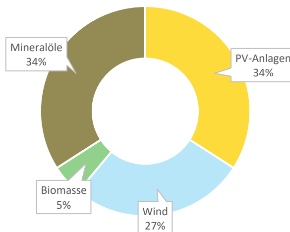
Abbildung 33: Anteile der vorhandenen lokalen Stromerzeugungsanlagen
