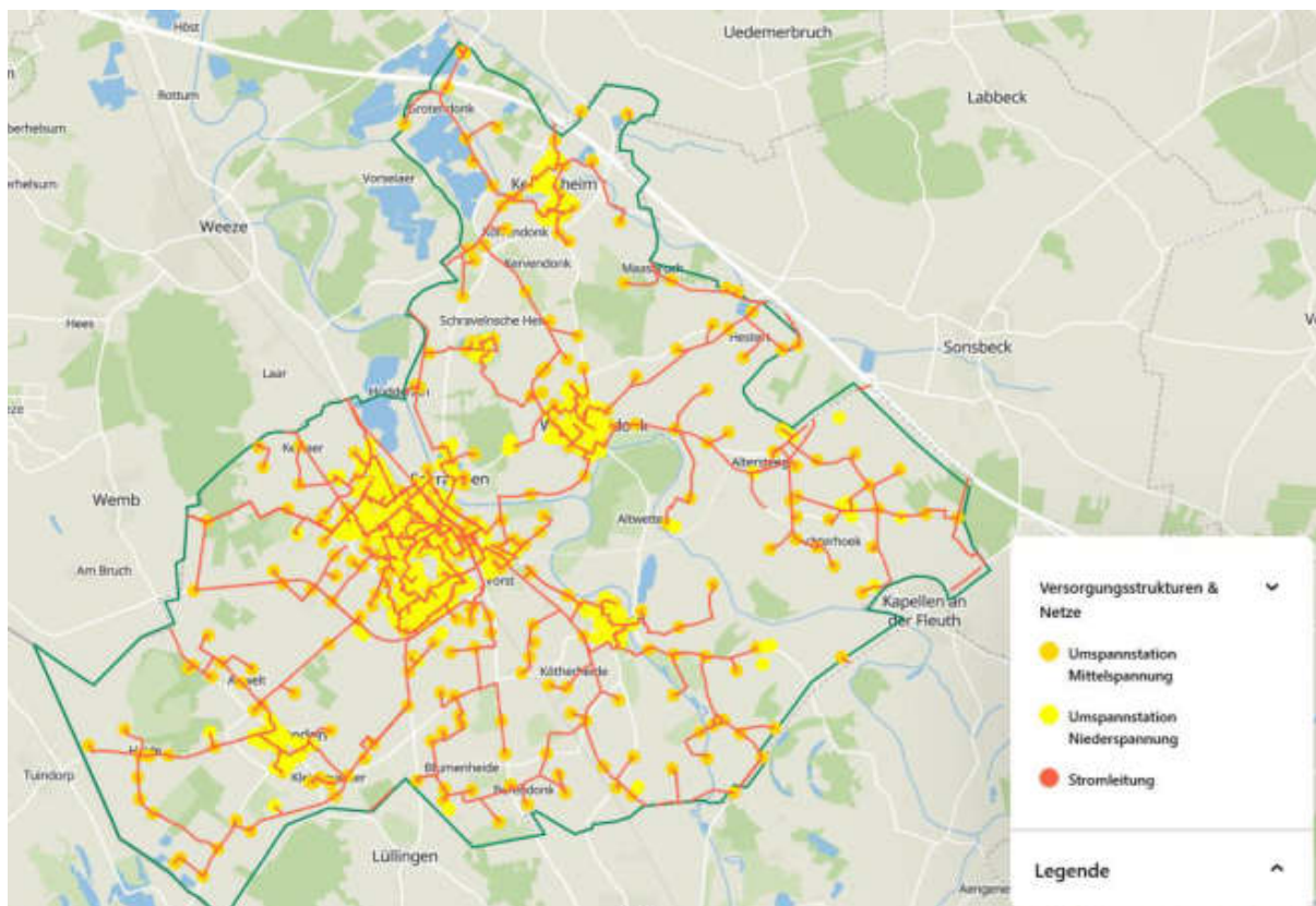
Abbildung 38: Stromnetze in Kevelaer auf Hoch- und Mittelspannungsebene einschließlich der Umspannstationen auf Mittelspannung und Niederspannung. Quelle: digitaler Zwilling (digipad)
