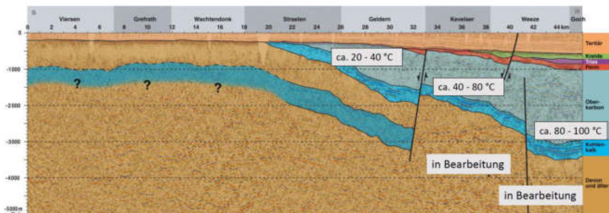
Abbildung 52: Darstellung der geologischen Perioden mit Temperaturniveau für die Wallfahrtsstadt Kevelaer [11]
