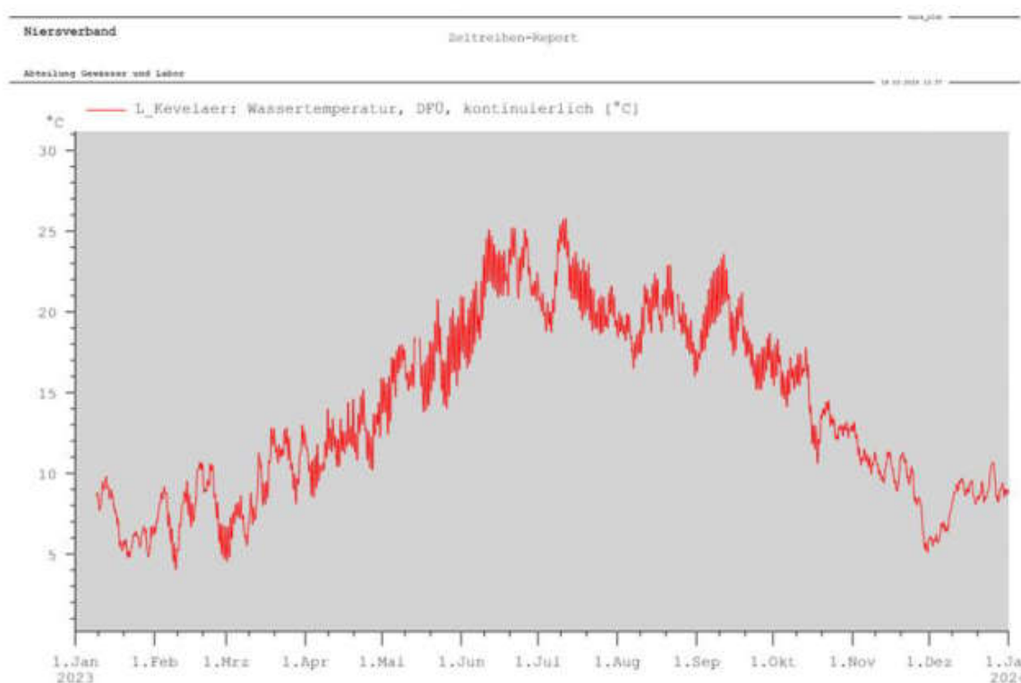
Abbildung 53: Temperaturprofil der Niers in Kevelaer. Quelle: Niersverband
