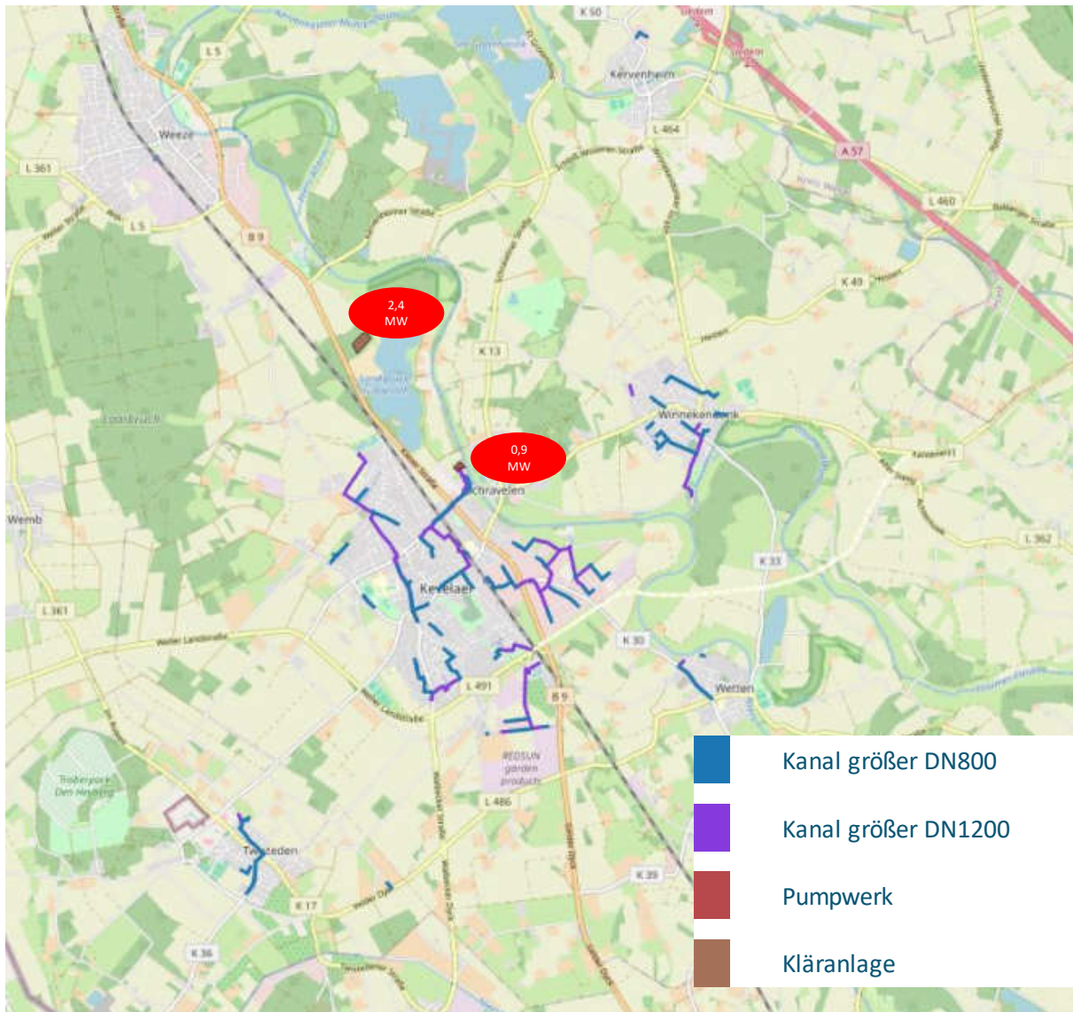
Abbildung 57: Darstellung des Kanalnetzes in Kevelaer mit >DN800 sowie Betriebsstätten
