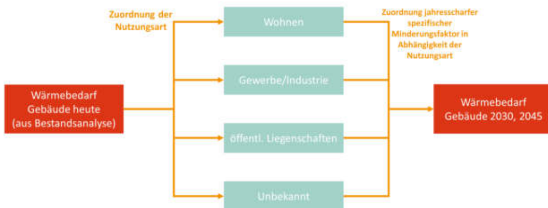
Abbildung 39: Vorgehen zur Ermittlung der Energieeinsparpotenziale
